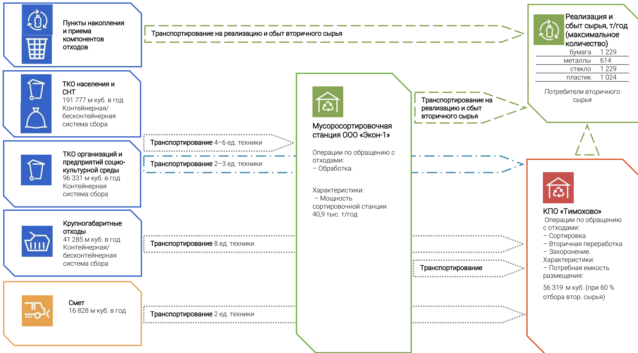
Рисунок 3.1.а – Предлагаемая логистика движения потоков ТКО, КГО и смета (показатели на 2020–2021 годы)
