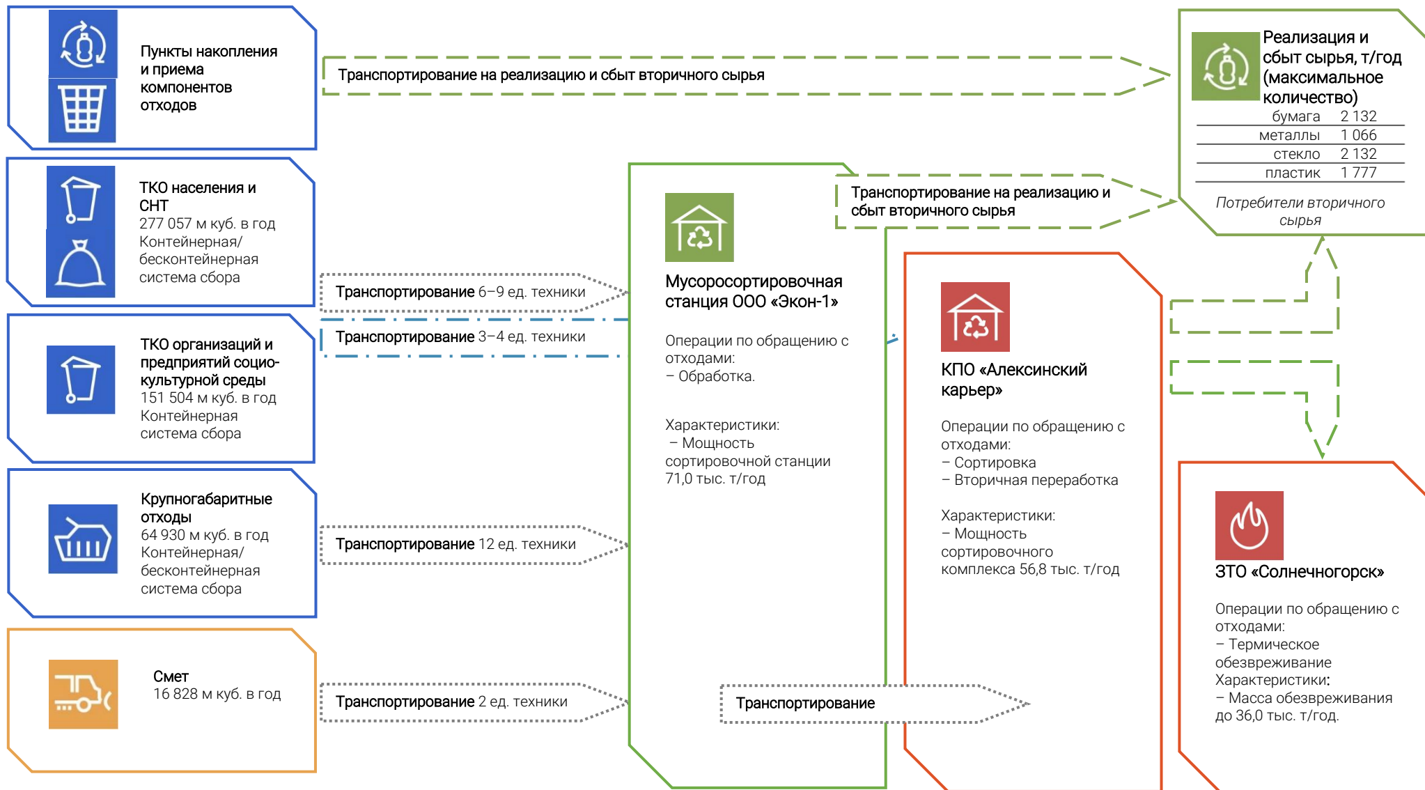
Рисунок 3.1.в – Предлагаемая логистика движения потоков ТКО, КГО и смета (показатели на 2035 год)
